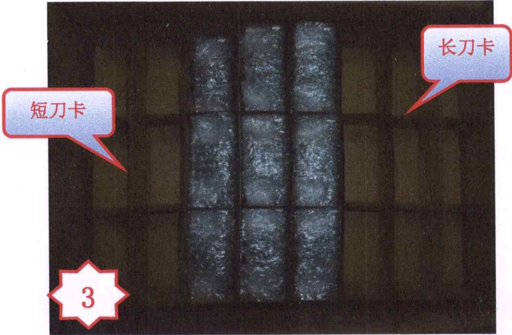
图三，将 PA1106 按照每层 144 个，每箱三层的方式进行包装，同时在底层和每层的顶部各放一块隔板，共 4 块隔板。
